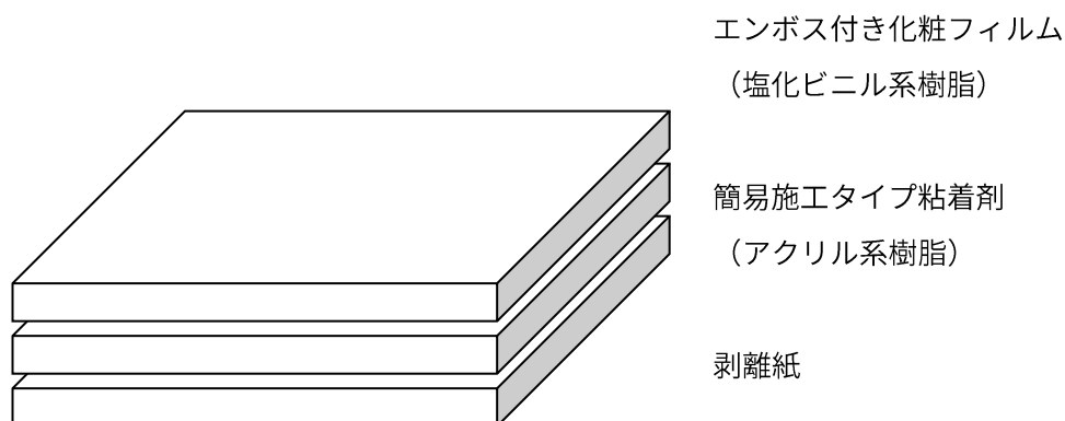
図 1 製品の構造
